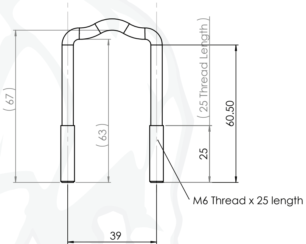
C064 U - Bolt M6 x 39 x 72
